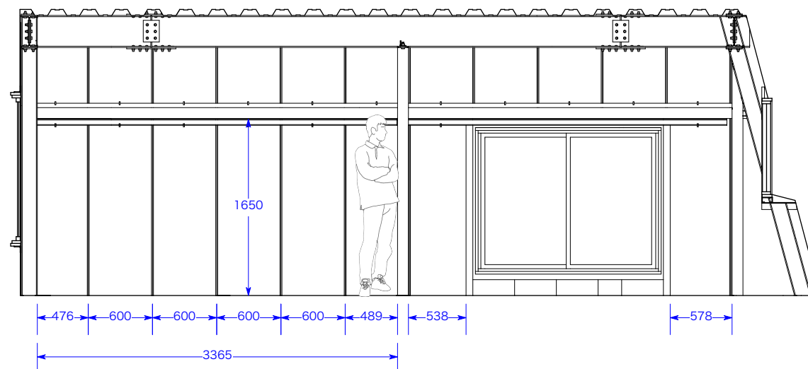
展開図 E (北側ALC壁)
