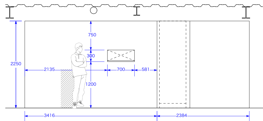
展開図 C (箱正面)
