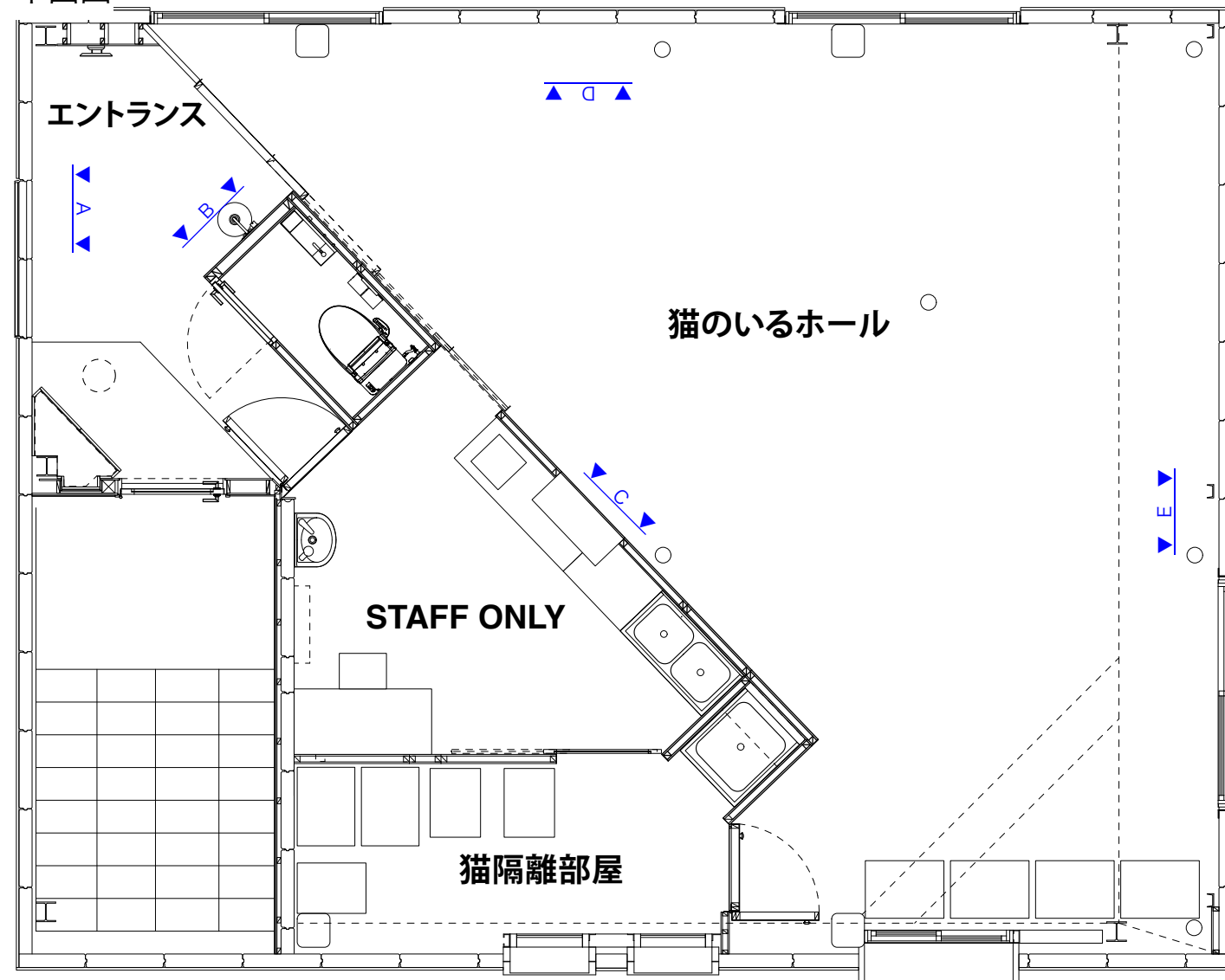
平面図
