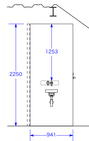
展開図 B (玄関手洗)
